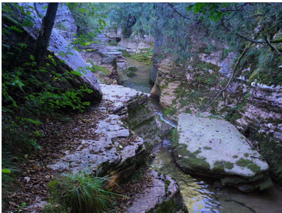
Vedute del Canyon di Cornolade. Fonte: Panoramio
